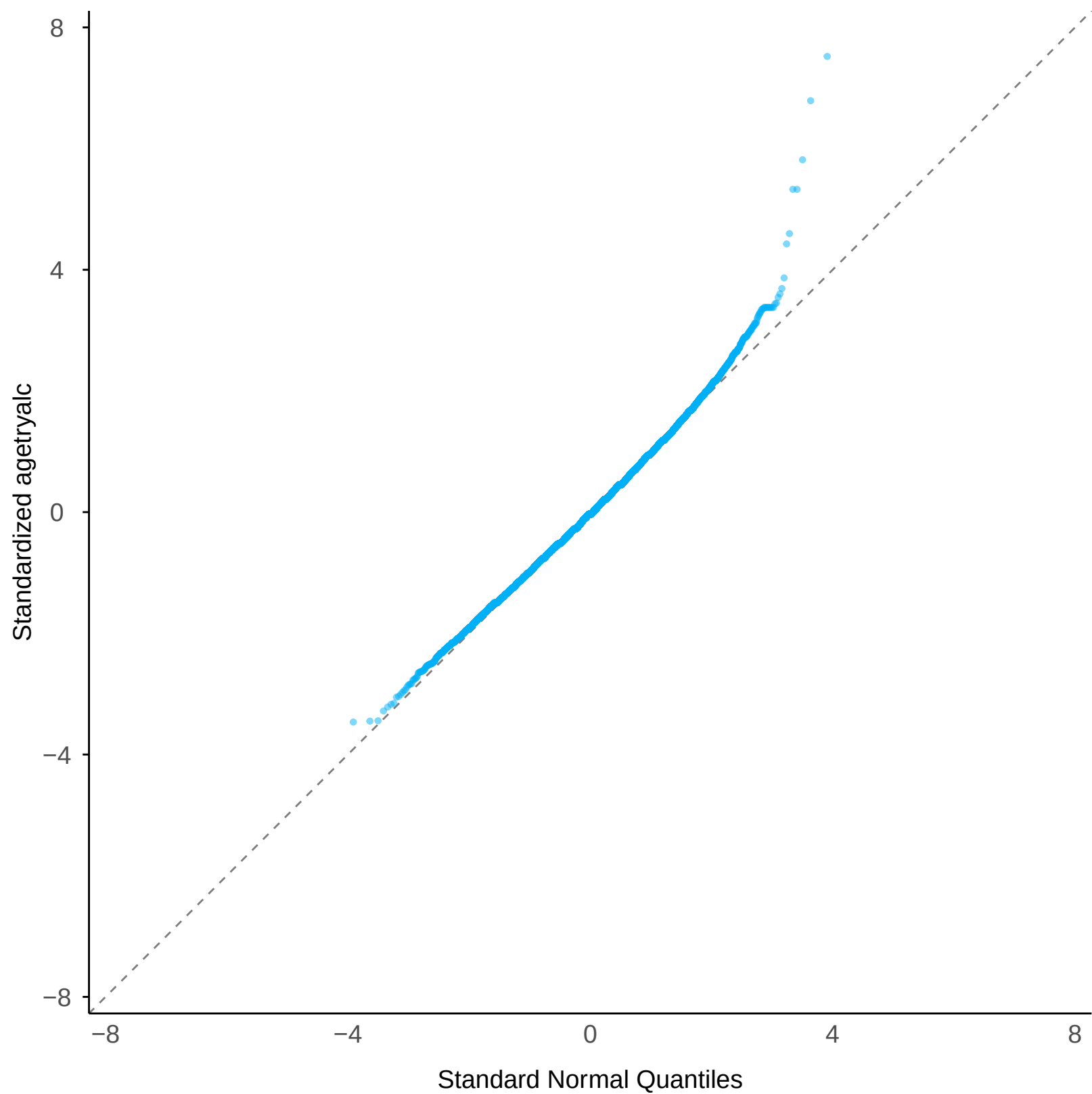
Normal Q-Q: agetryalc
